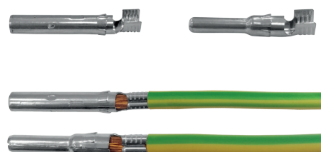
Pressform des Kabelschuhs an der Leitung
