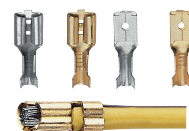
Форма обжима наконечника на проводе.
