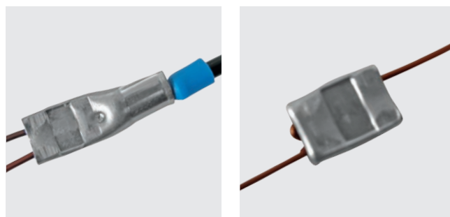
Форма опрессовки разъема на проводе.
