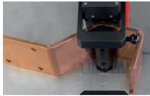
Biegen HG 201.
