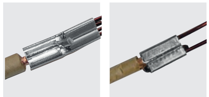
Forma zaprasowania złączki na przewodzie.
